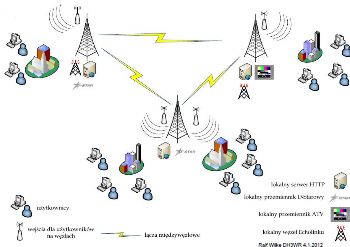
Rys. 1.2.1. Struktura sieci
