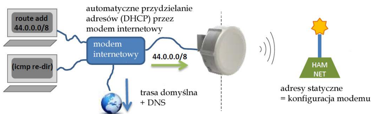
Rys. 1.2.3. Zasada konfiguracji sieci domowej dla integracji Hamnetu z Internetem (źródło: http://routerboard.com )
