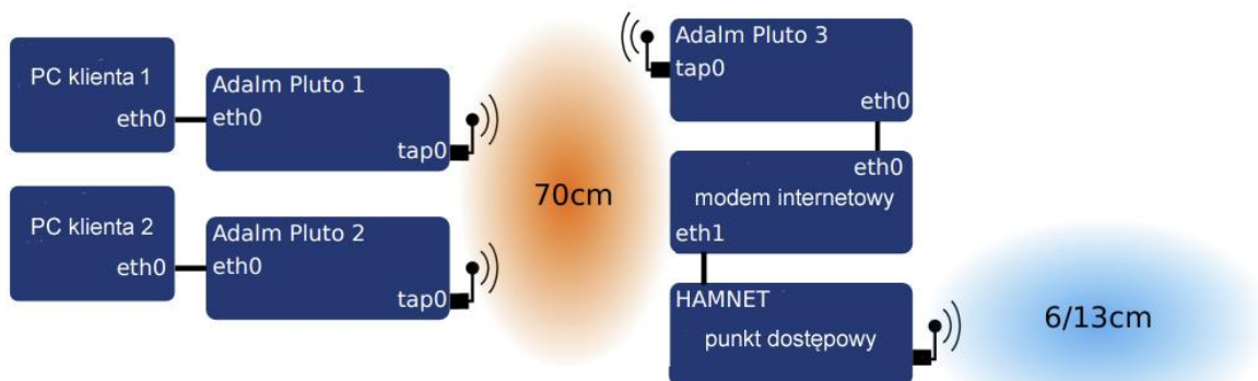
Rys. 10.1.2. Połączenie pojedynczej stacji z punktem dostępowym
